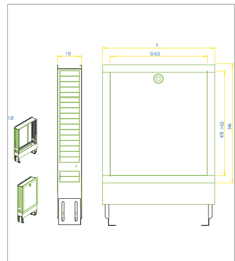
armario xFlat planos de montaje y plantillas CAD disponibles
